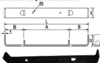
Ecarteur de pied de banche
